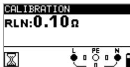
Weerstand van de meetkabels voor de compensatie.
