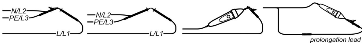
Kortgesloten meetkabels
