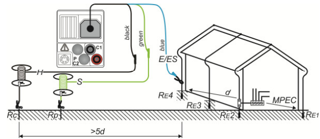
Aansluiting van de als optie verkrijgbare aardingsset (044113)
