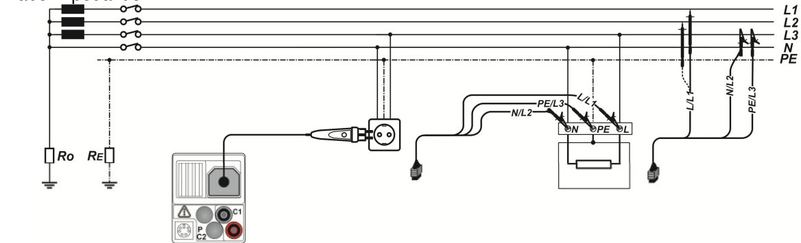
Aansluiting van de als optie verkrijgbare Commander meetstekker (044149) en de 3-aderige meetkabel
