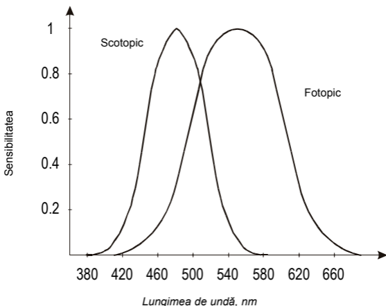
Figura 3: V(\lambda) curba pentru sensibilitatea ambelor situații
