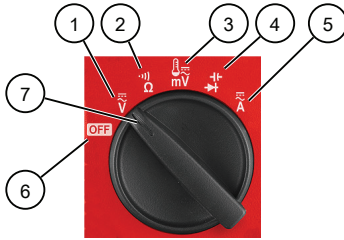
Afbeelding 7: Draaischakelaar
