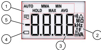
Afbeelding 8: Digitaal display
